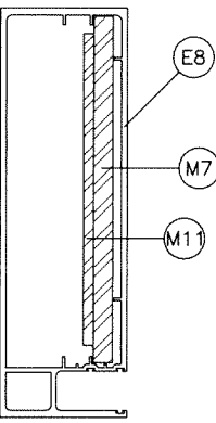
JAMB 'J3'
