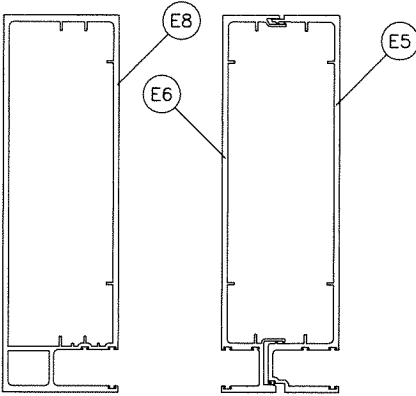
JAMB 'J1' MULLION 'M1'
